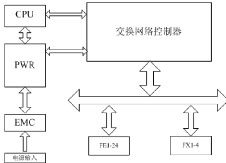
图 3-1 WitNet IAS3028A 硬件结构图
